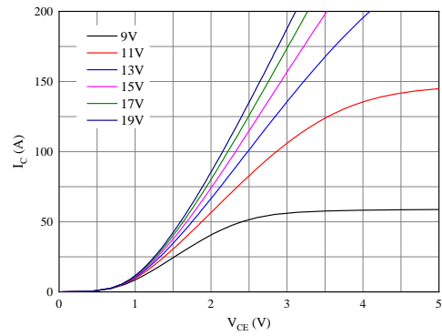
图 2. 典型输出特性 ( T_{vj}=150°C )
